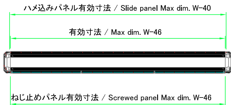
A-A ( 1 : 8 )
